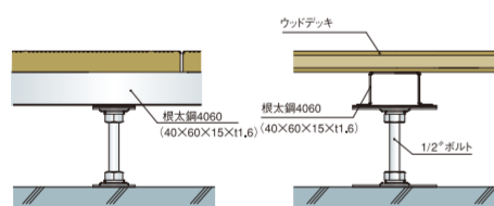
根太シングル工法断面図
