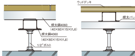
根太クロス工法断面図
